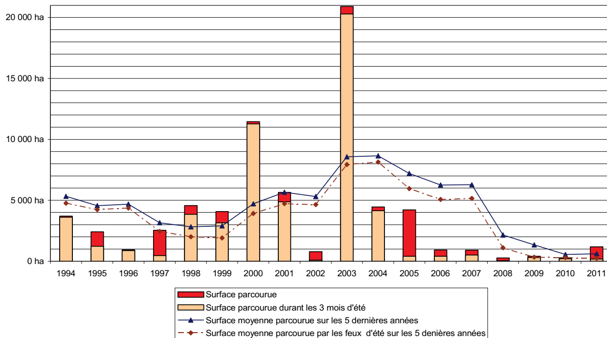
HAUTE CORSE : Surface parcourue par les feux (données Prométhée 1994-2011)
